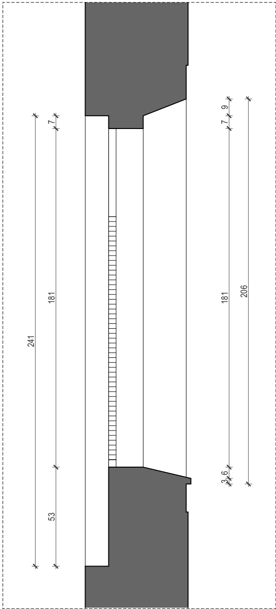
presjek prozora zvonika
