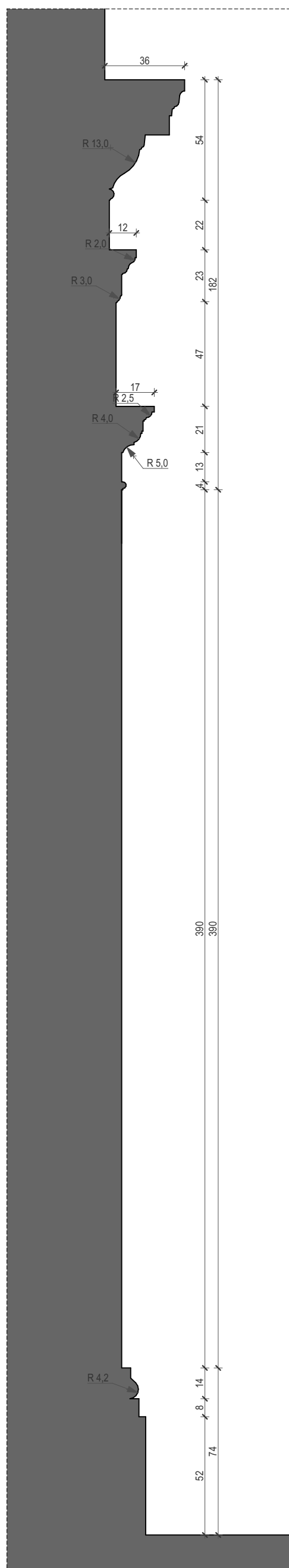
presjek unutarnjeg vijenca crkve na stupu
