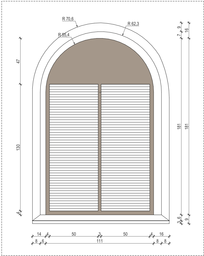
pogled prozora zvonika
