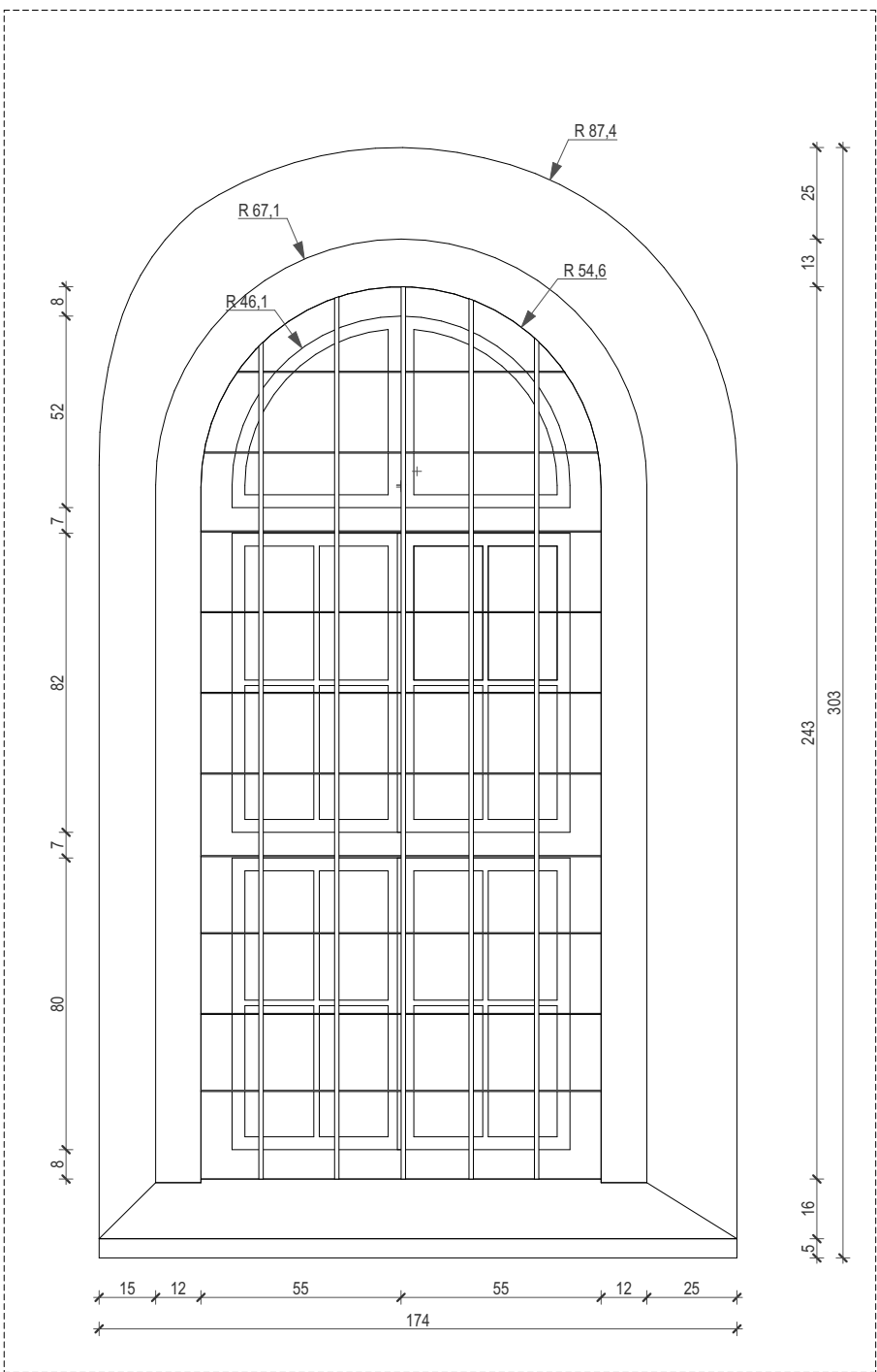
pogled prozora crkve
