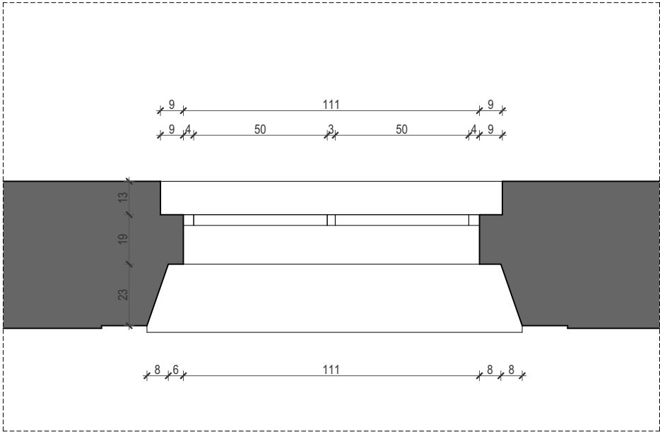
tlocrt prozora zvonika
