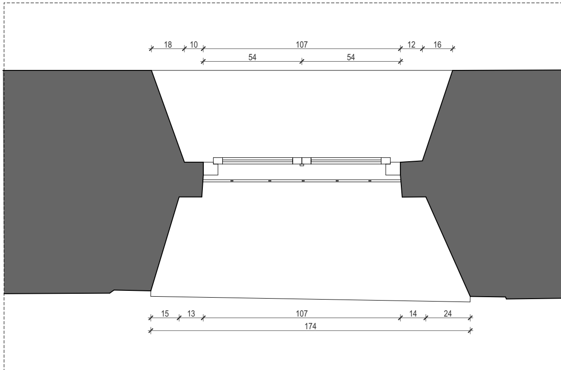
tlocrt prozora crkve
