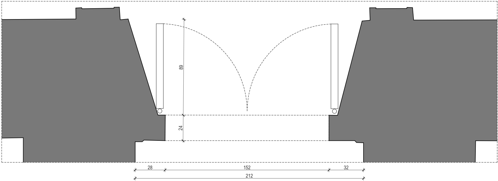
tlocrt ulaznih vrata
