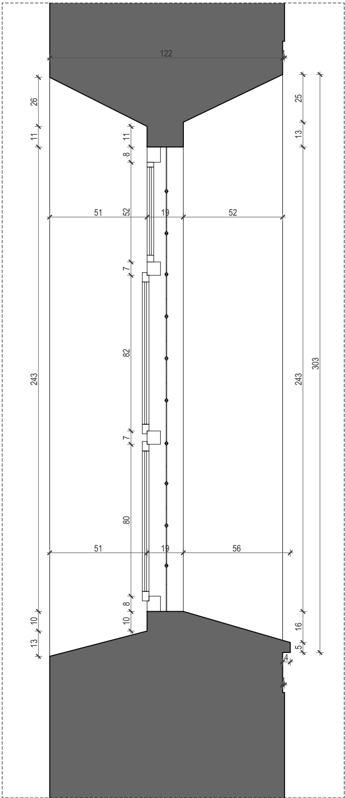
presjek prozora crkve
