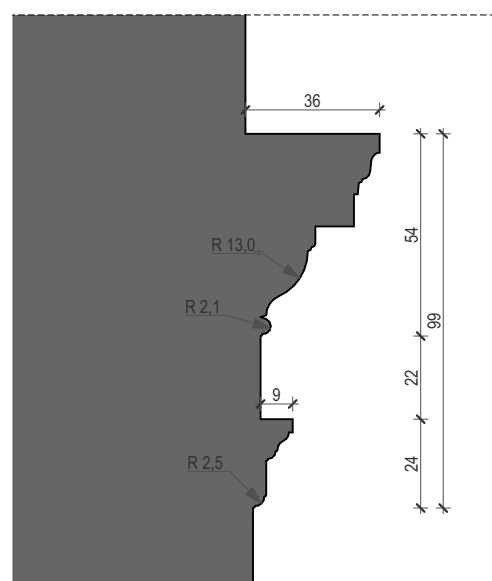
presjek unutarnjeg vijenca crkve na zidu
