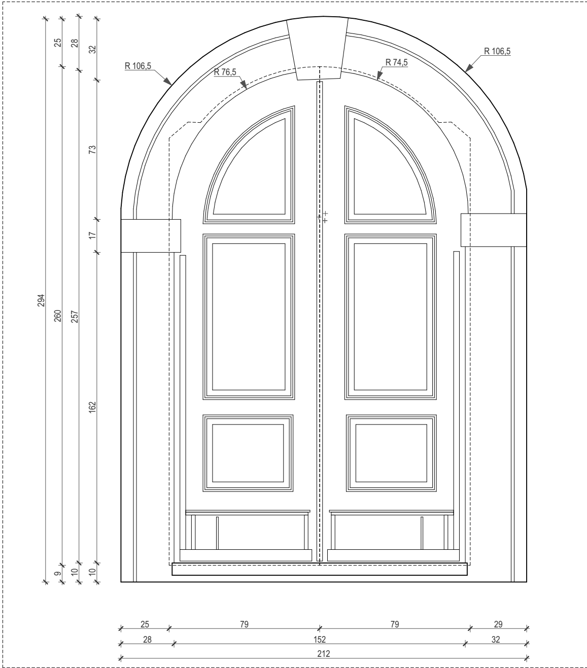
pogled ulaznih vrata
