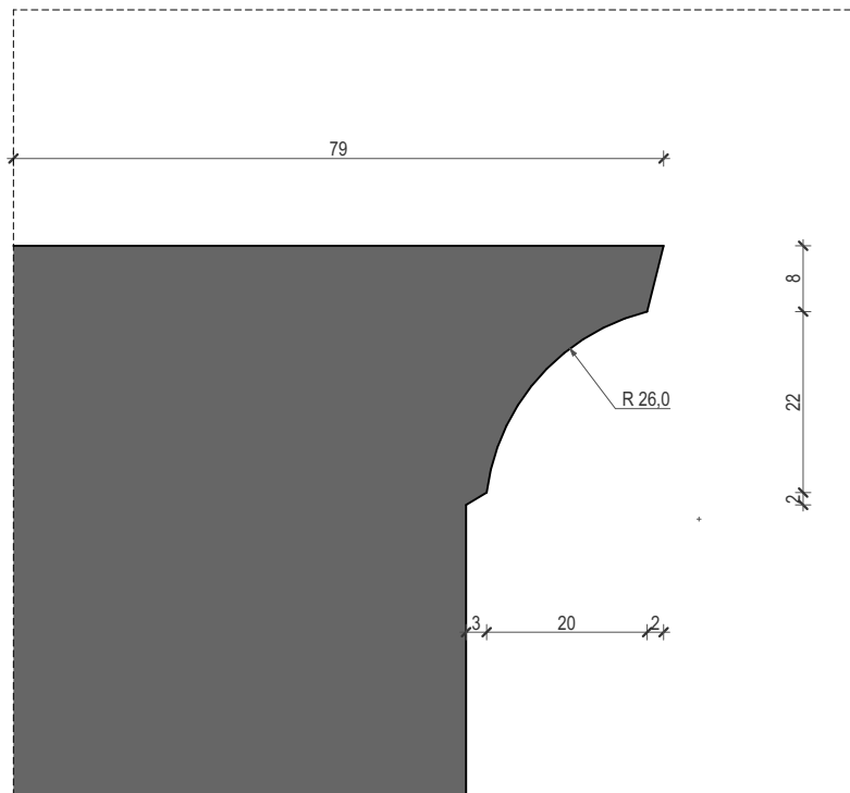
presjek vijenca zvonika
