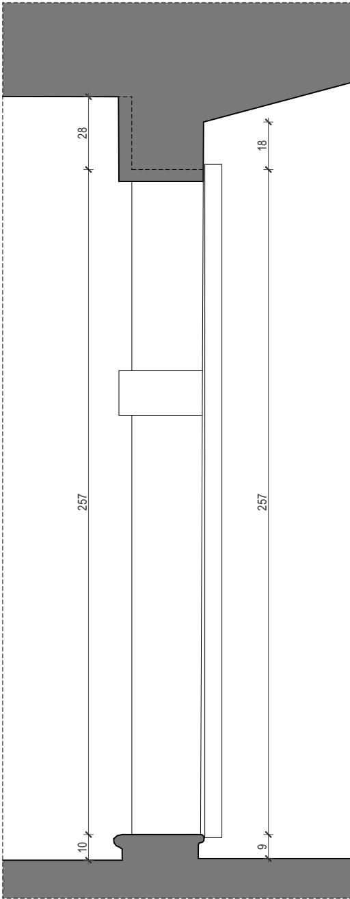
presjek ulaznih vrata
