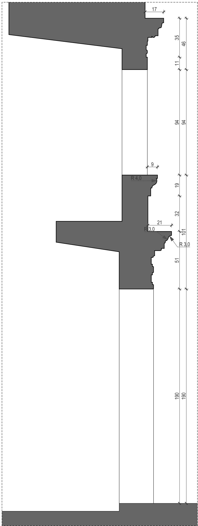
presjek ulaza u sakristiju
