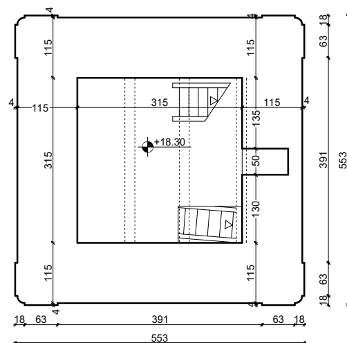
TLOCRT 5. KATA ZVONIKA
