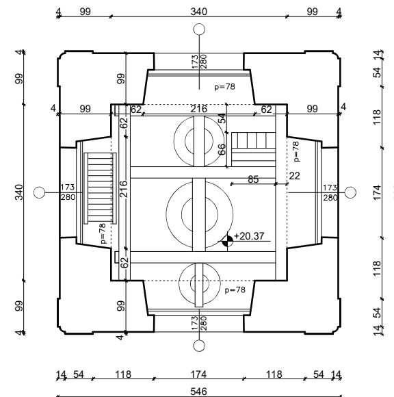
TLOCRT 6. KATA ZVONIKA
