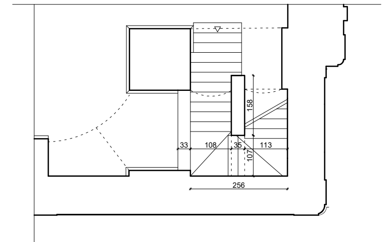
TLOCRT STUBIŠTA NA KOR
