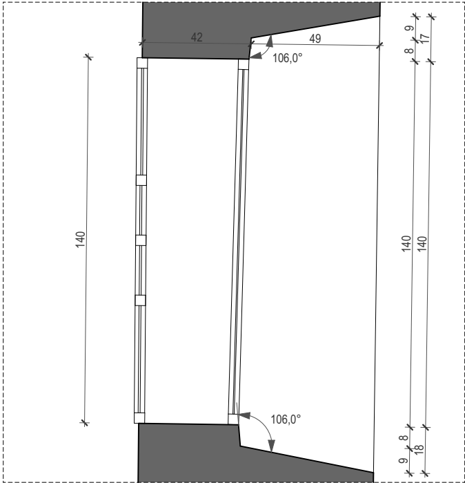
tlocrt prozora crkve
