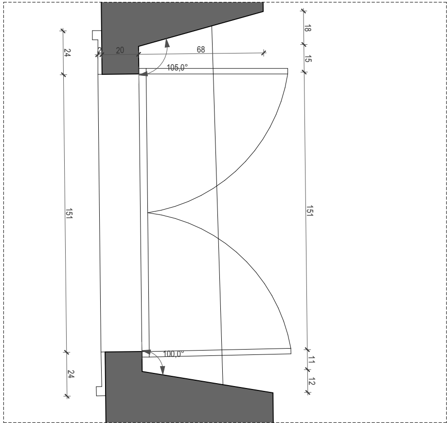
tlocrt ulaznih vrata
