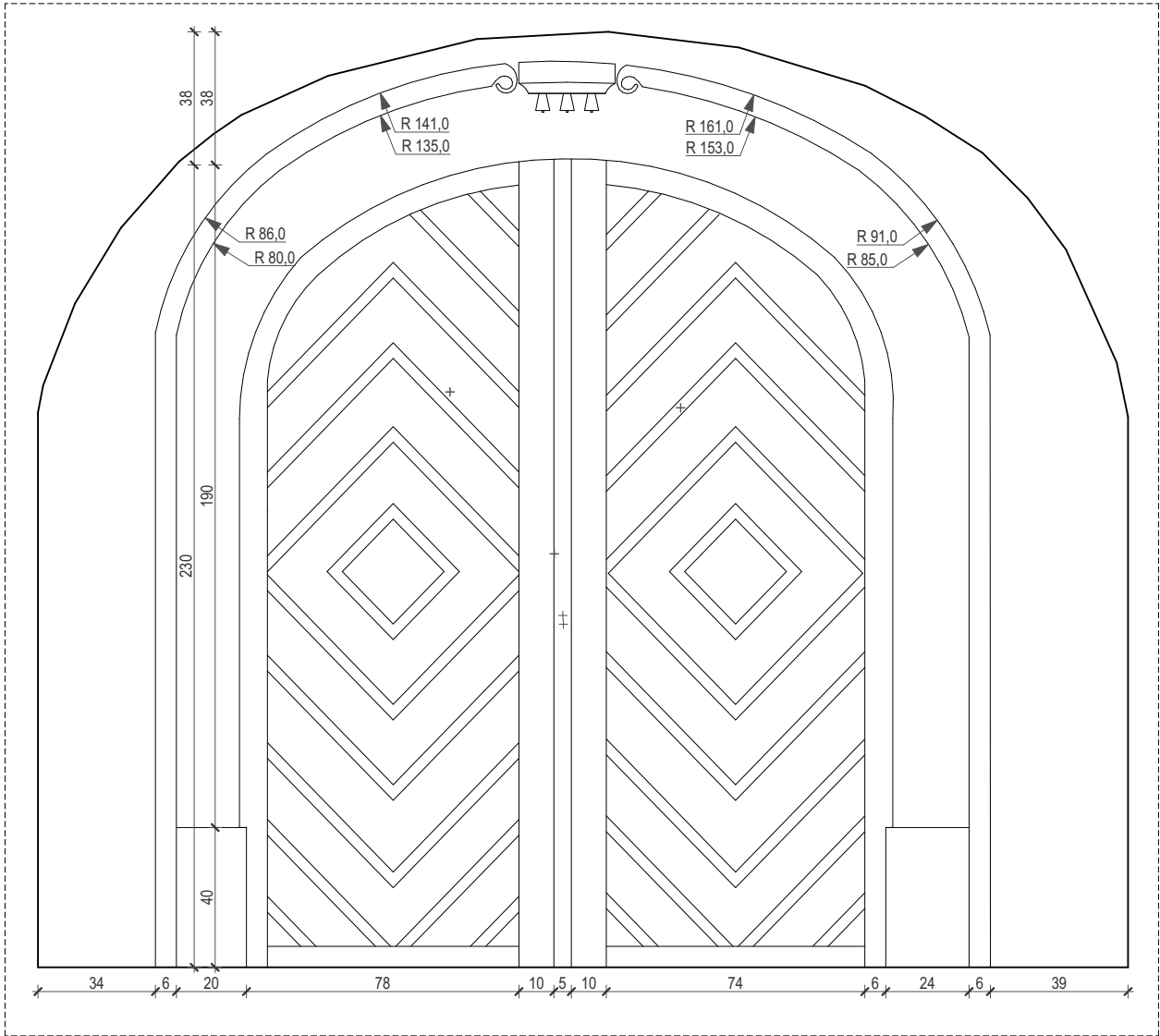
pogled na ulazna vrata
