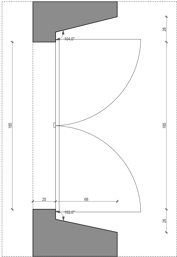
tlocrt ulaznih vrata
