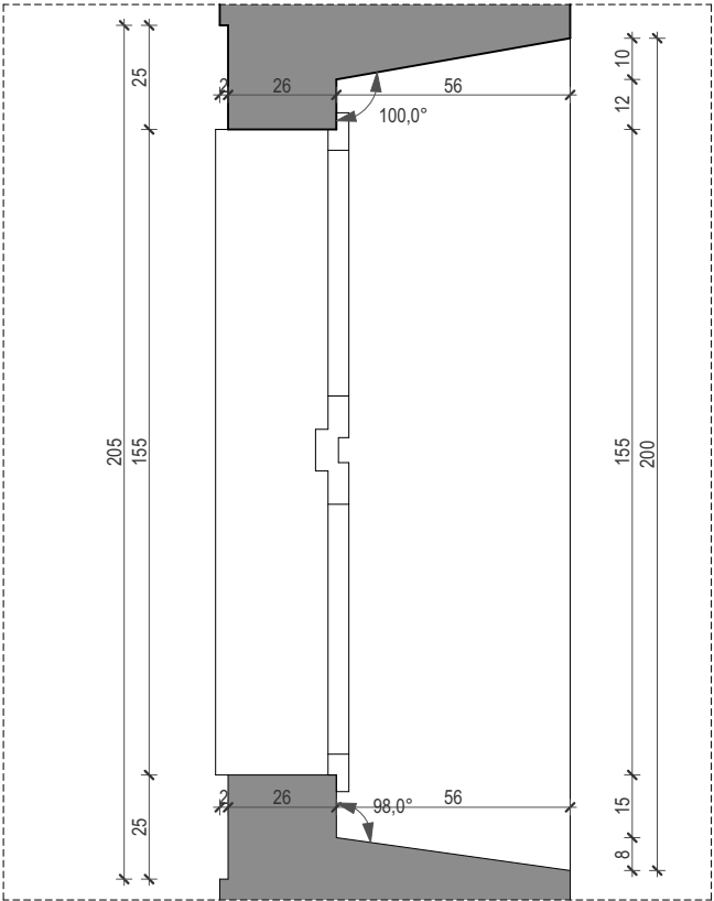
tlocrt prozora zvonika
