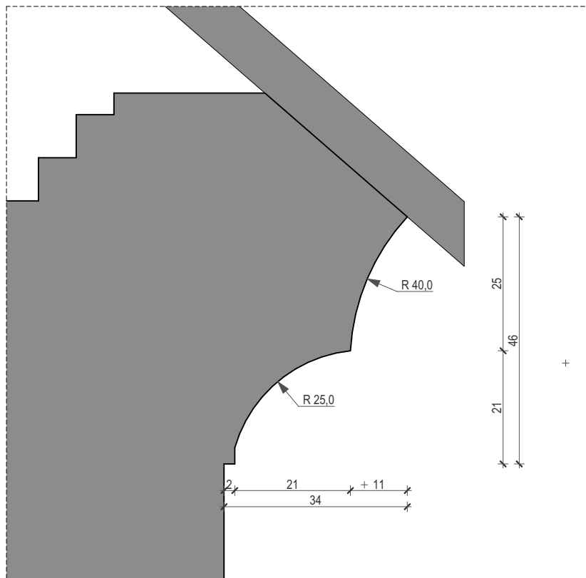
detalj vijenca crkve
