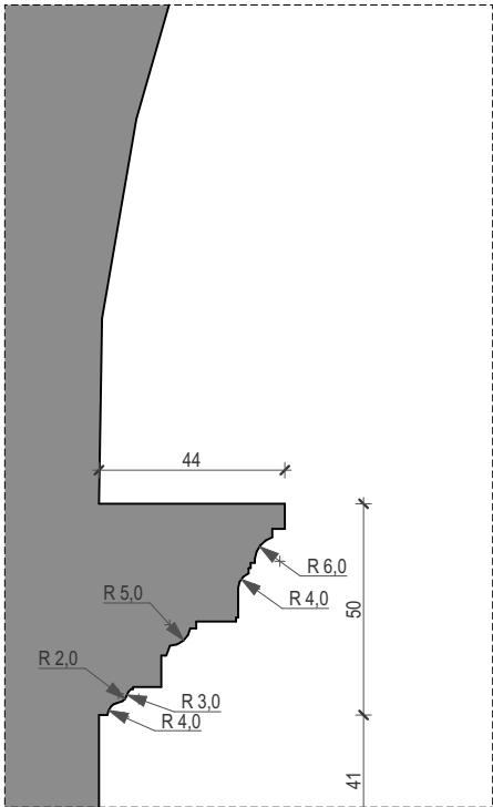
detalj profilacije na stupu
