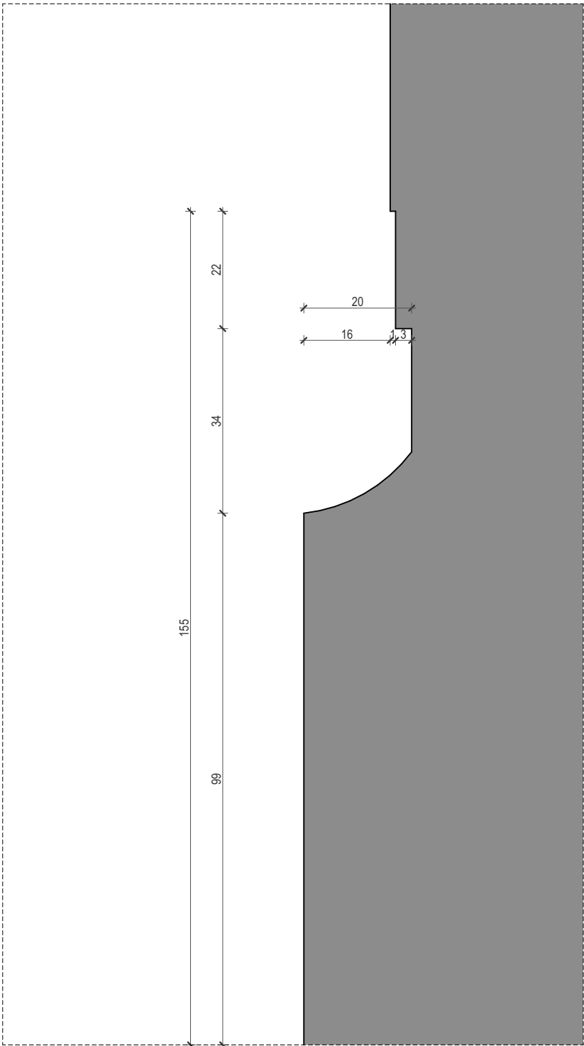
detalj sokla
