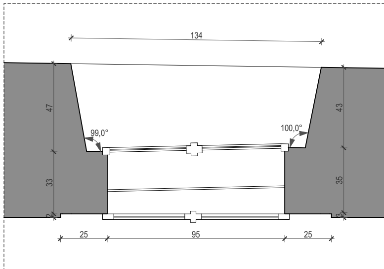
tlocrt prozora sakristije
