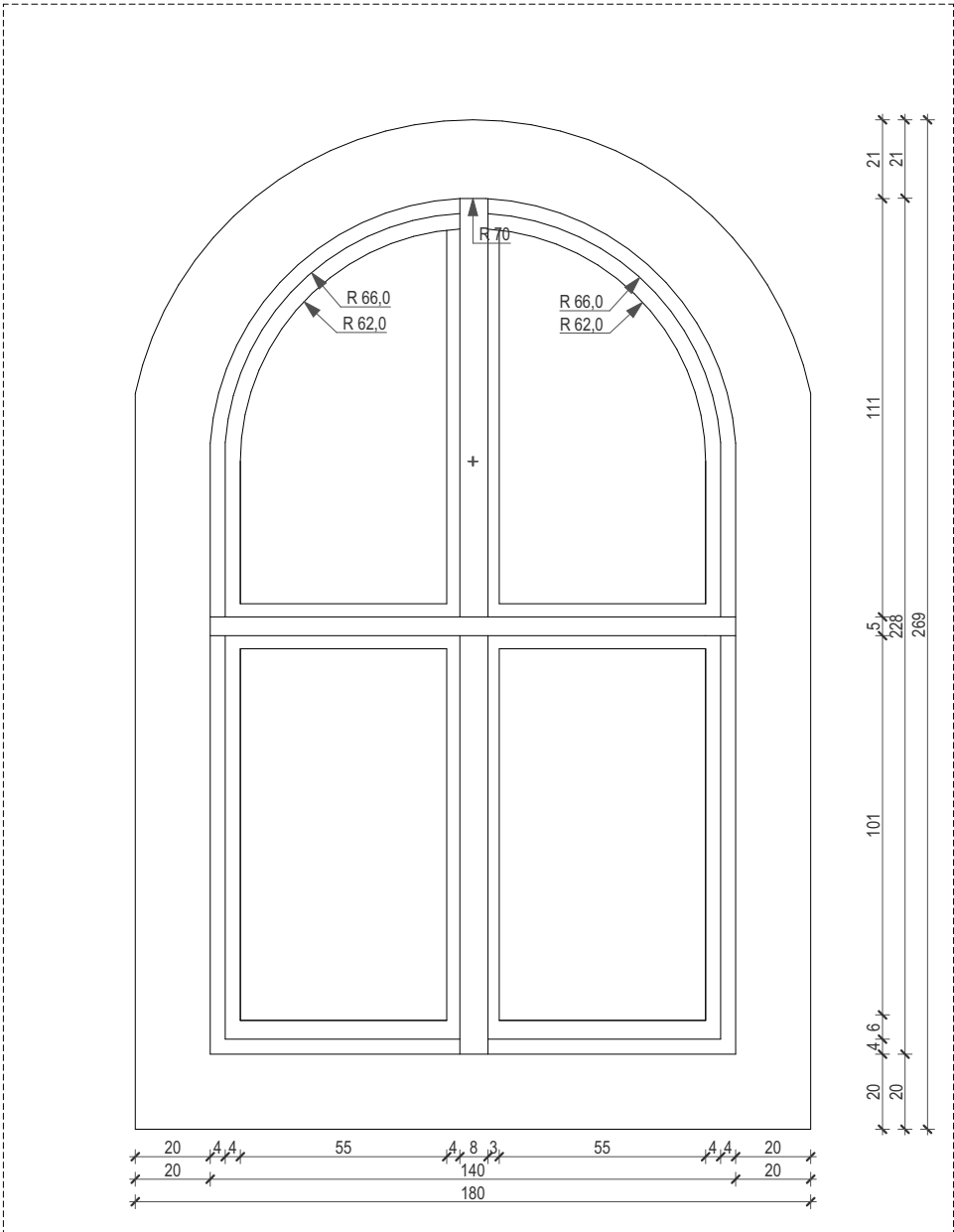
pogled na prozor crkve
