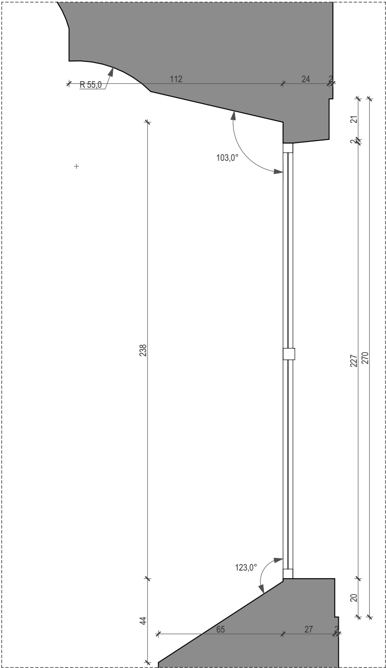
presjek prozora crkve
