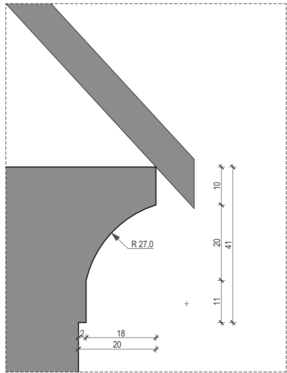
detalj vijenca sakristije
