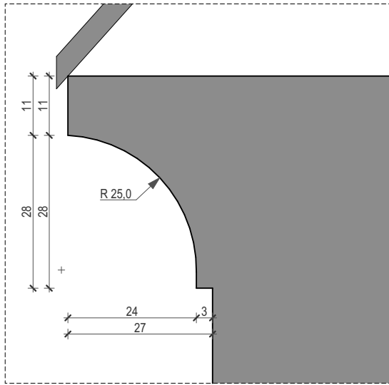
detalj vijenca - zvonik
