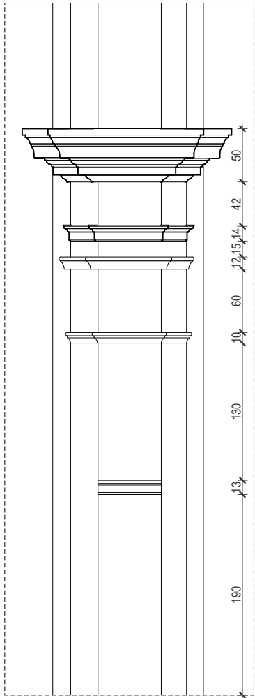
pogled na profilaciju stupa
