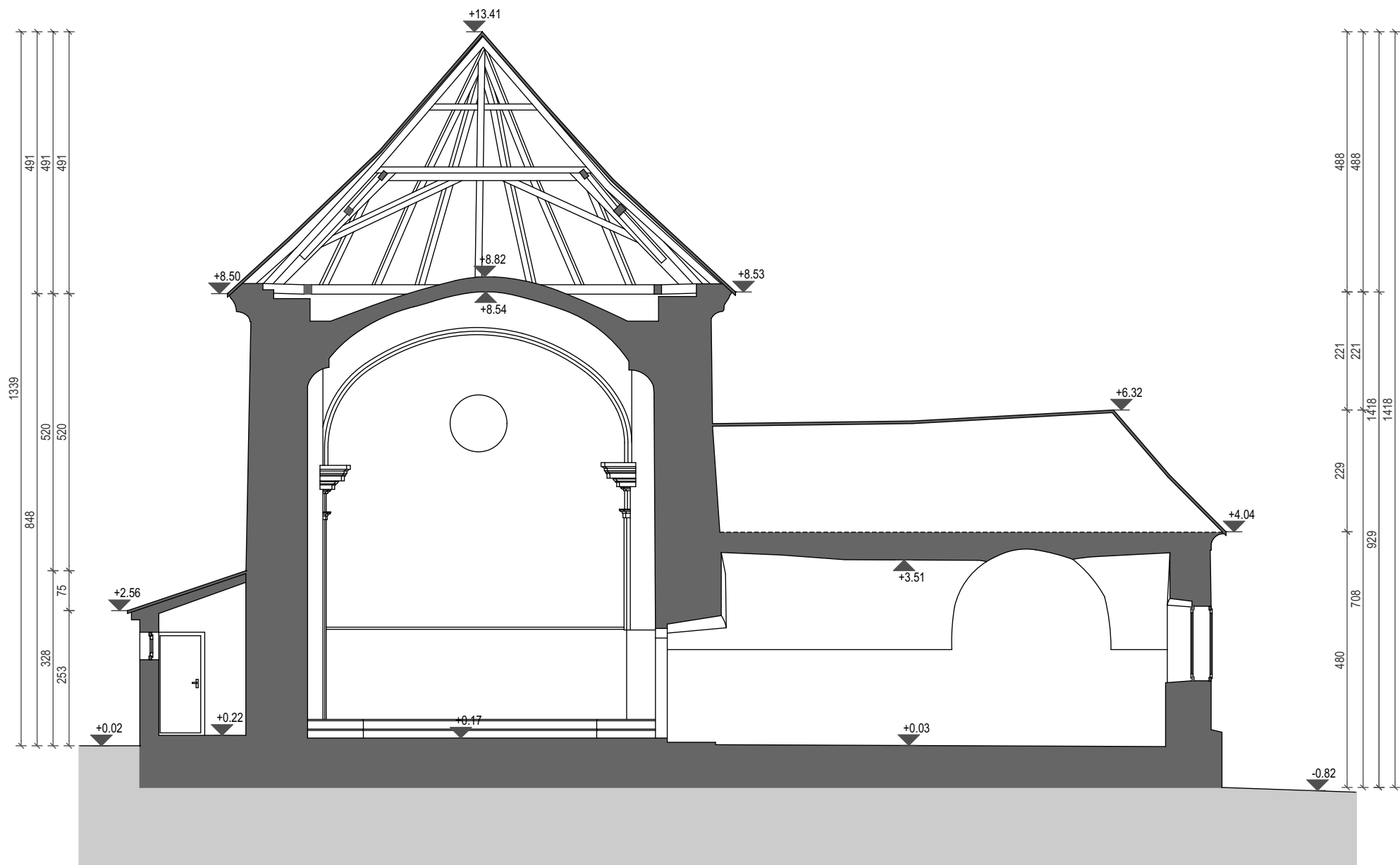
presjek C
